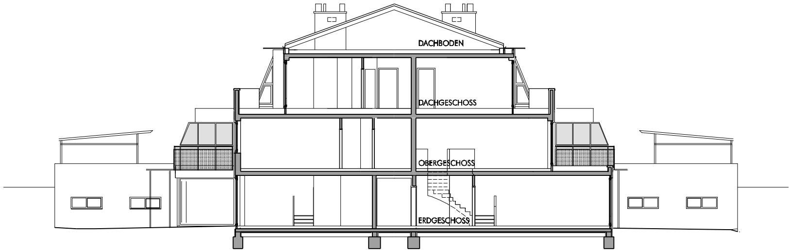
SCHNITT 2-2
