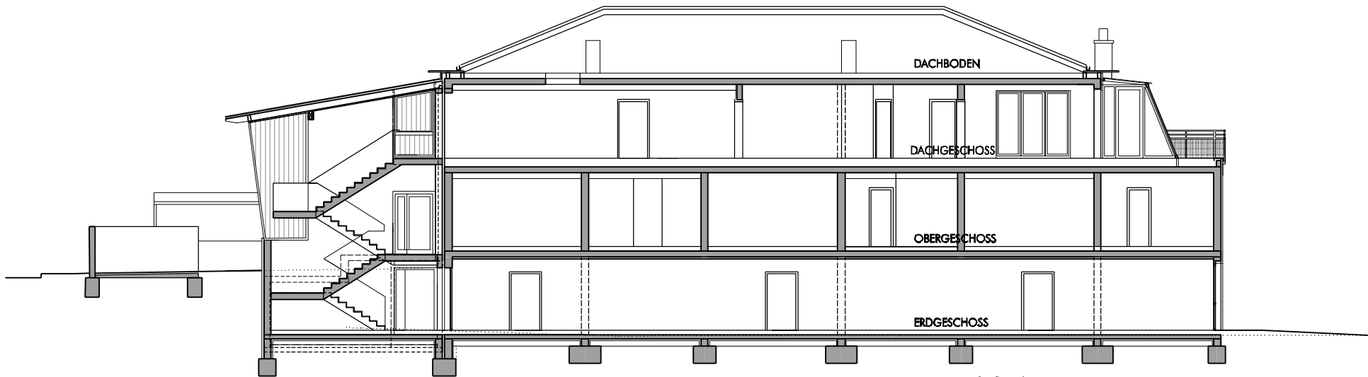
SCHNITT 3-3
